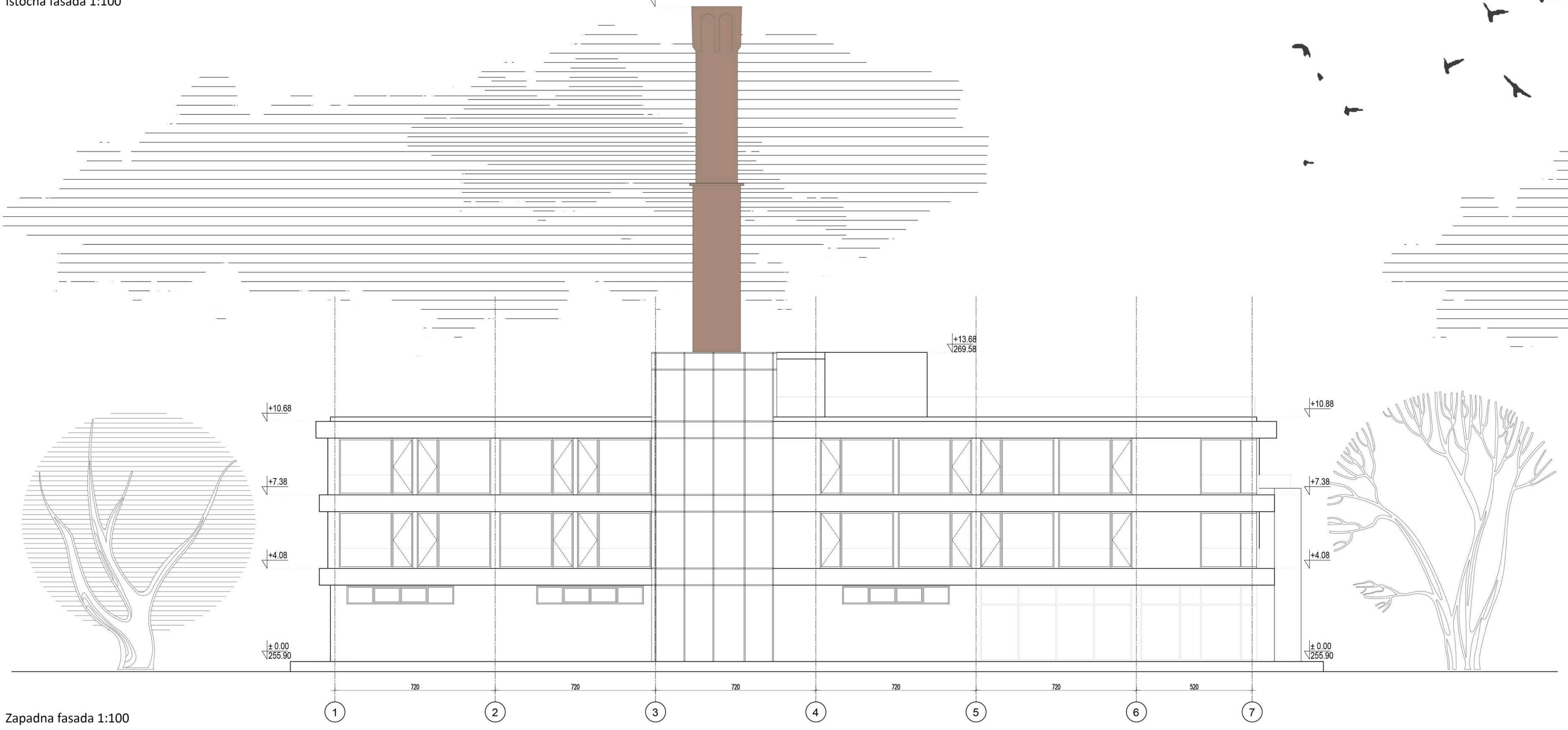
Zapadna fasada 1:100
