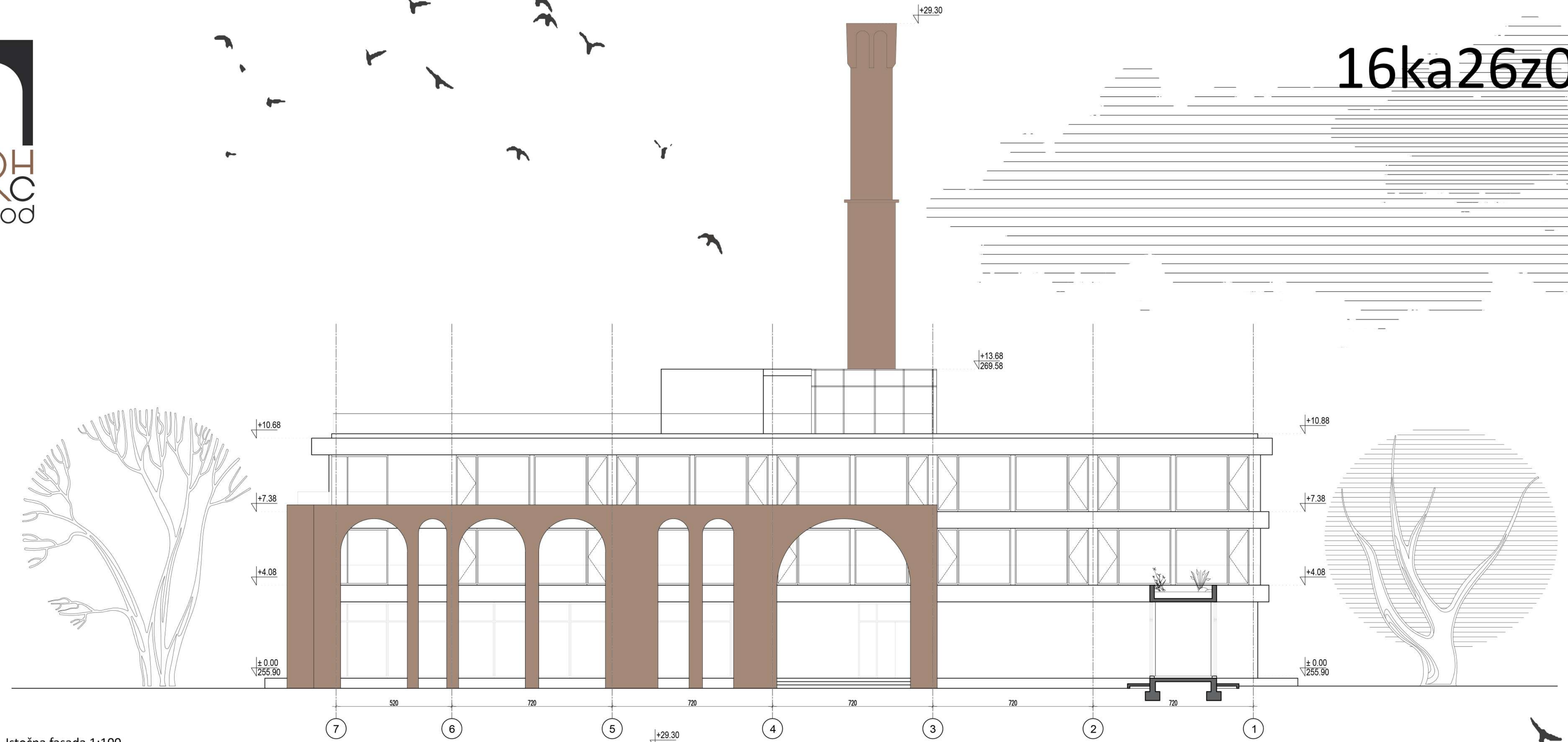
Istočna fasada 1:100
