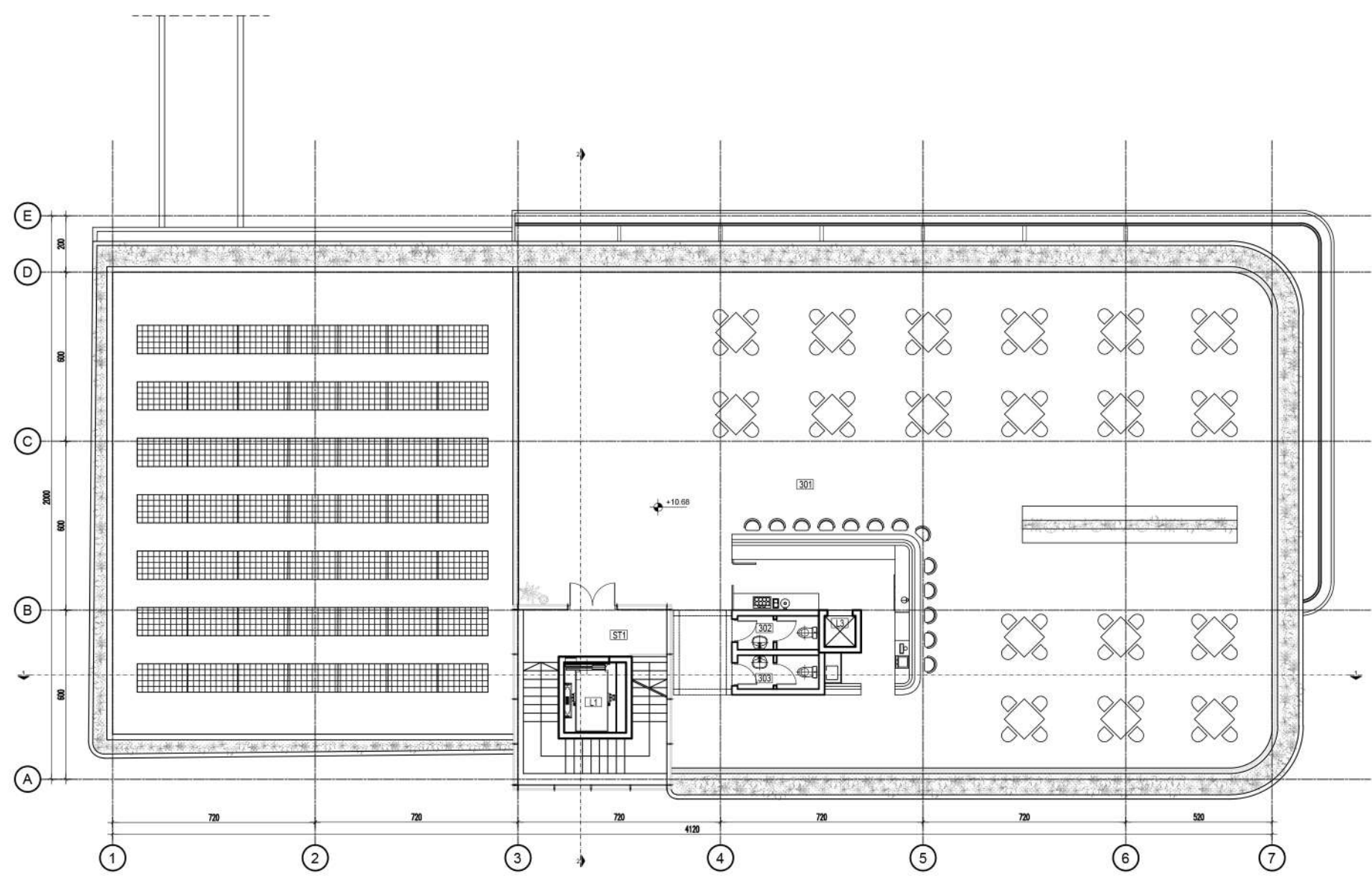
Osnova krova 1:200
