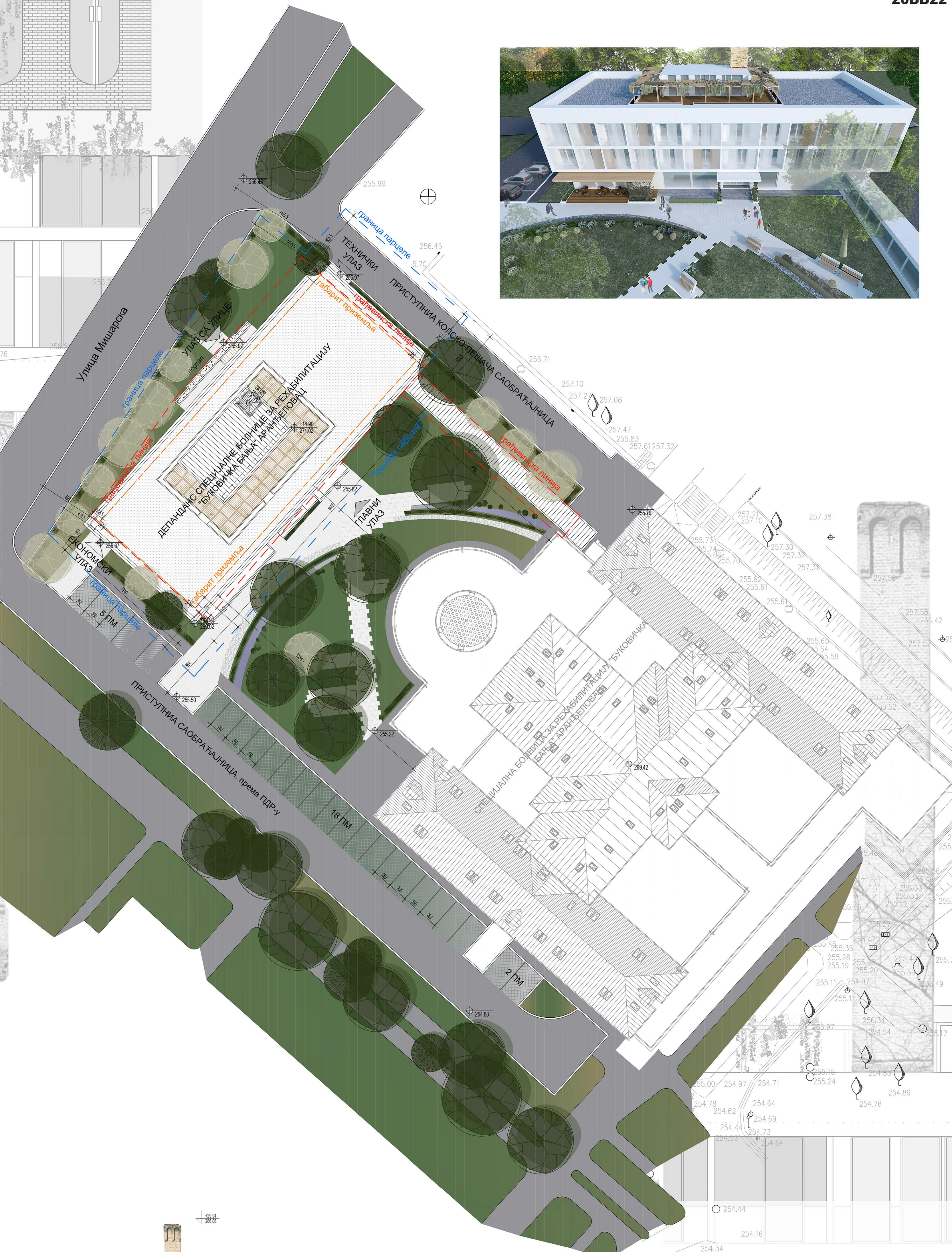
СИТУАЦИЈА - КОМПОЗИЦИОНИ ПЛАН P=1:200
